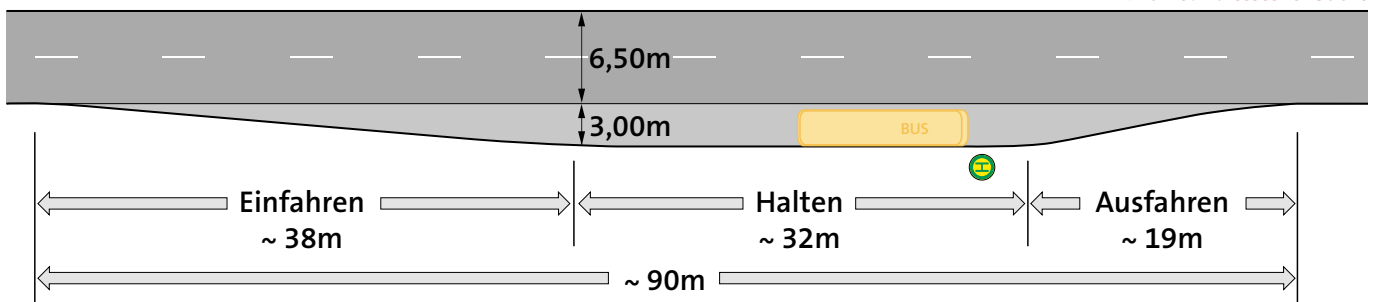
Bild 26: Haltestellenbucht
